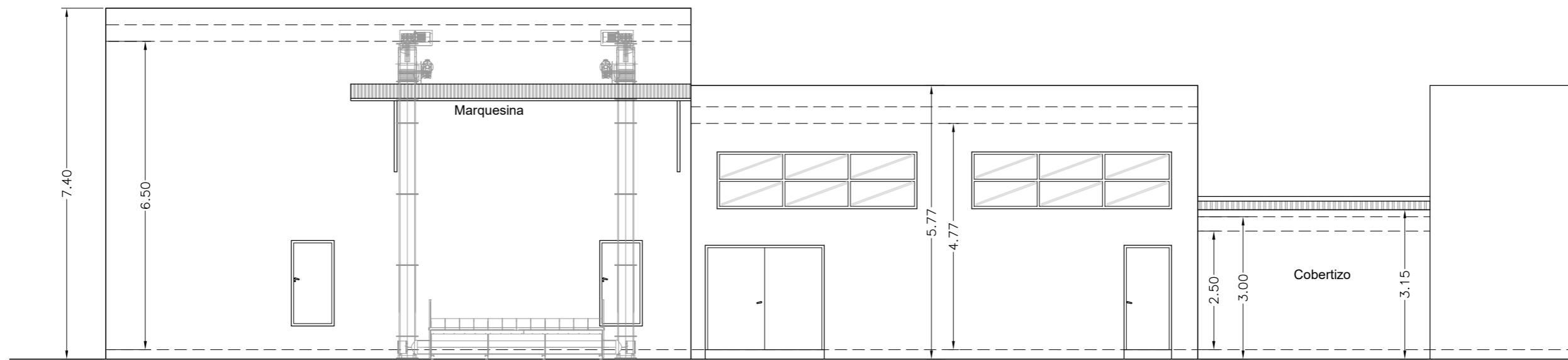
ALZADO SUR (OPCIÓN ACCESO A)
