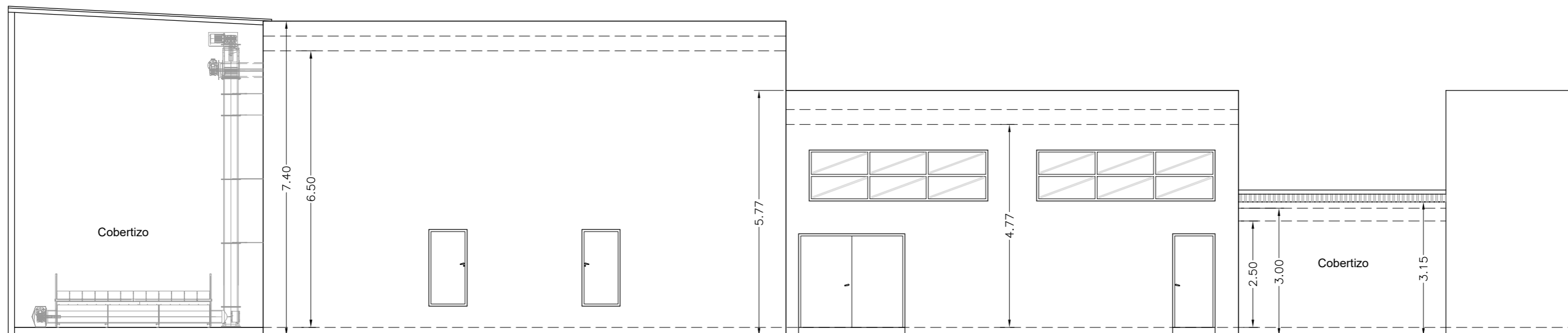
ALZADO SUR (OPCIÓN ACCESO B)
